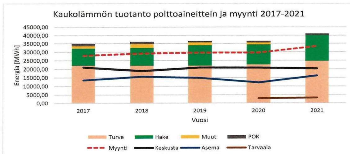
Kaavio 1. Kaukolämmön tuotanto polttoaineittain ja laitoksittain sekä myynti 2017-2021
