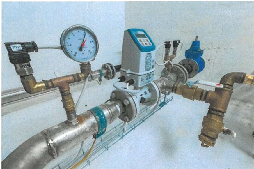
Kuva 2. Kalkanlahden saneerattu paineenkorotuspumppaamo
